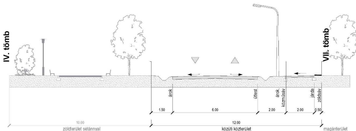
Mintakeresztmetszvény a keleti oldali út kialakításához
